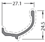
CODE / KOD 45T-501-00 THEORETICAL WEIGHT kg/m TEORİK AĞIRLIK kg/m 0.219
